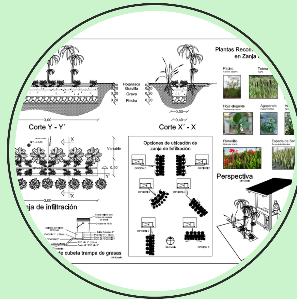
Projeto de diversos sistemas de tratamento e reuso de águas cinzas para uma ecovila. Local: México.
