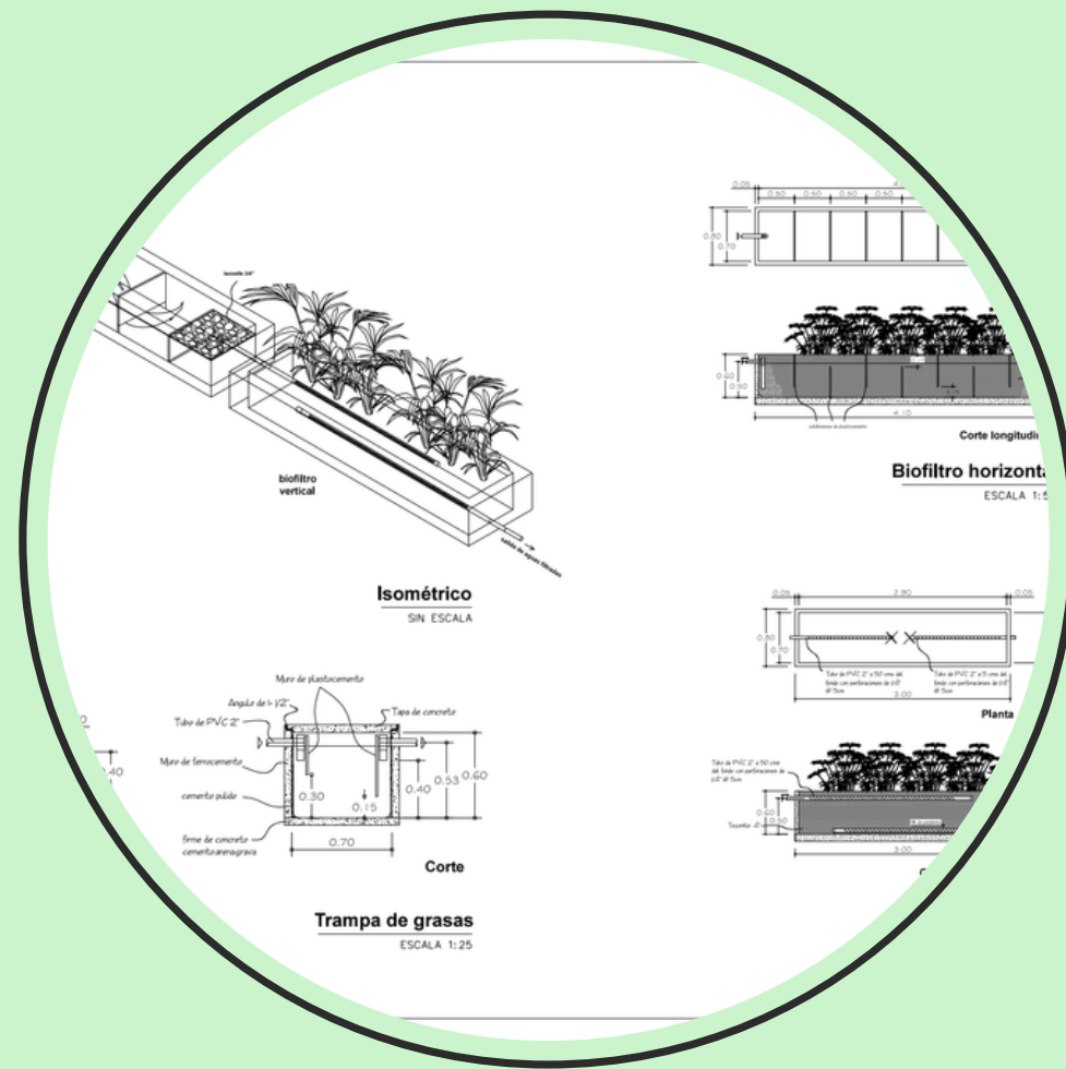
Projeto de zona de raízes de fluxo horizontal e vertical para uma casa de duas pessoas. Local: México.
